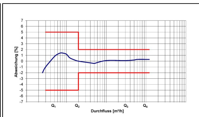
Typische Fehlerkurve
