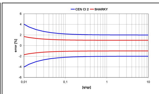
Courbe enveloppe
