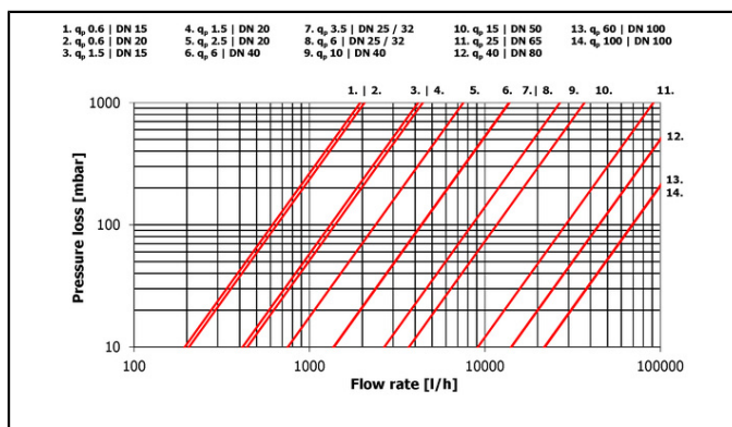
Tryktabskurve
