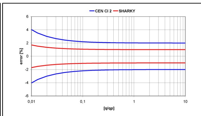
Typisk fejlcurve
