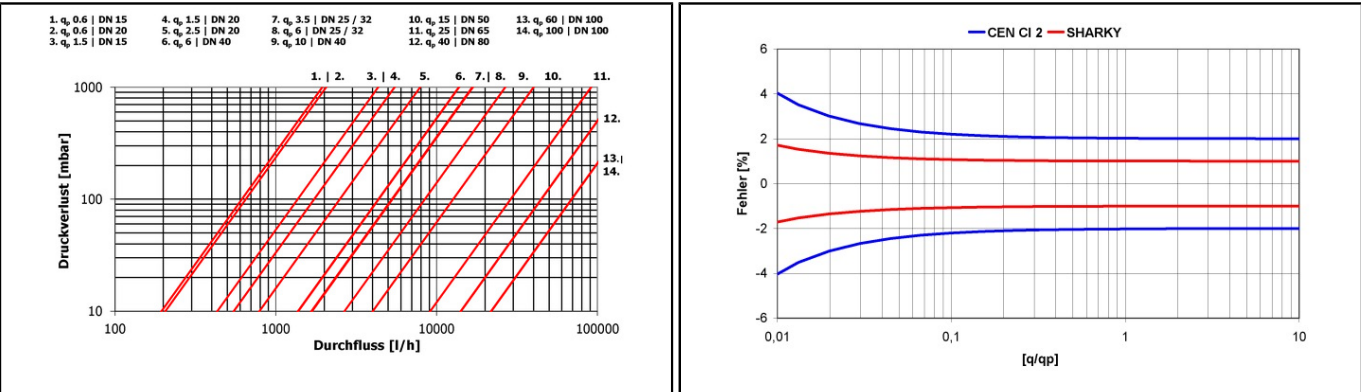
Druckverlustkurve
