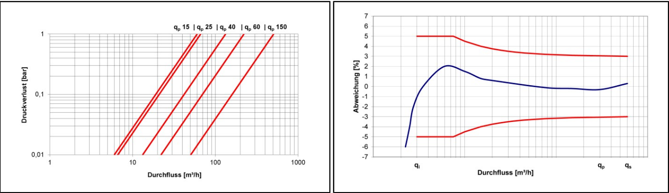
Druckverlustkurve
