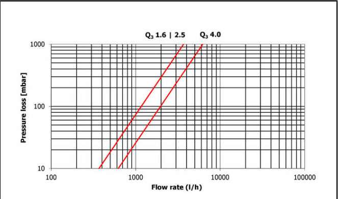
Tryktabskurve
