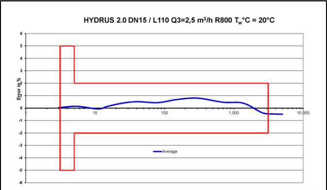
Typische Fehlerkurve
