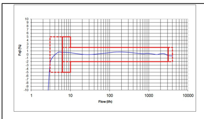
Typisk fejlkurve
