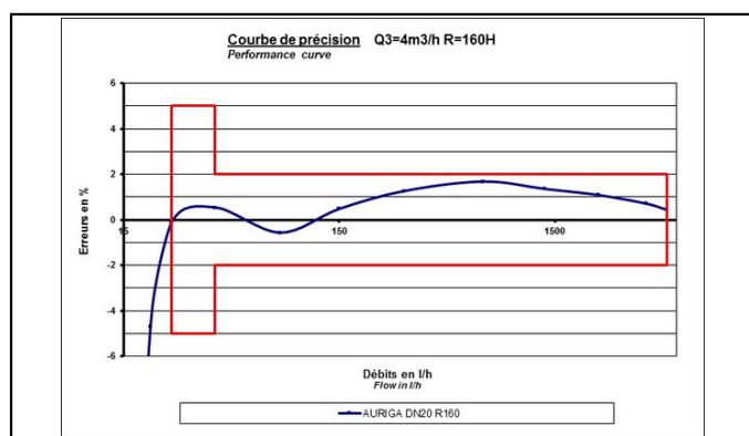
DN20 - Mosiądz
