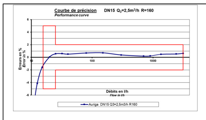
DN15 - Mosiądz
