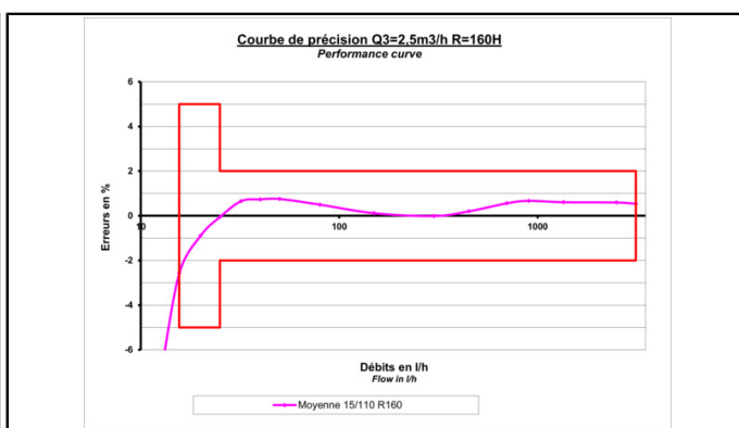
DN15 - Kompozyt
