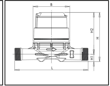
DN 20 Kunststoff
