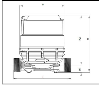
DN 15 Kunststoff
