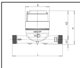
DN 20 laiton
