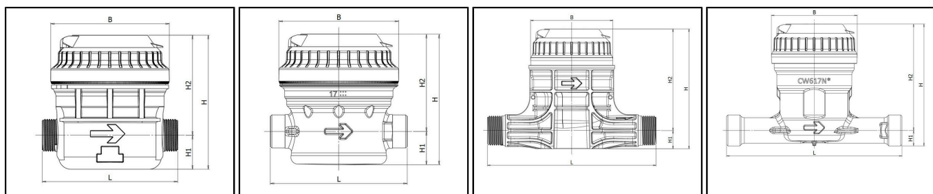
Seitenansicht DN 15 (Kunststoff) DN 20 - Messing
