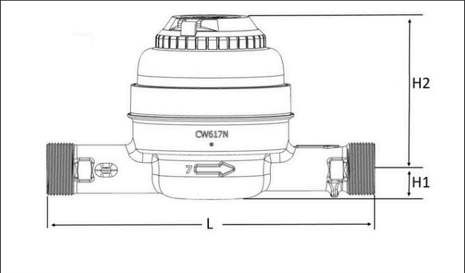
Vue de face - DN40
