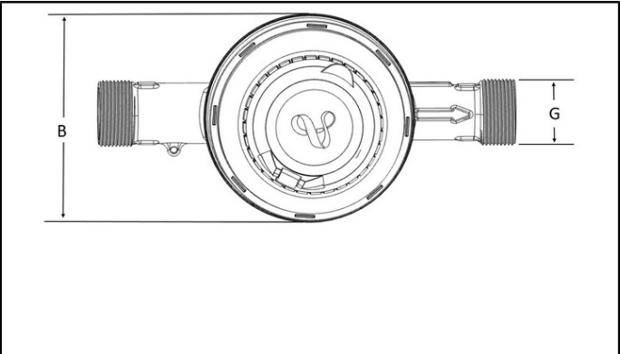
Draufsicht
