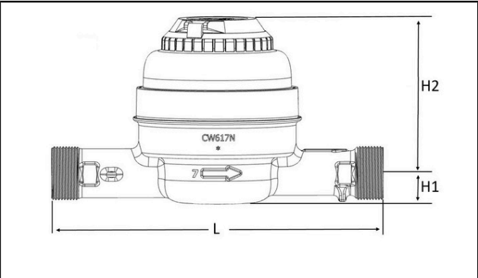
Frontansicht - DN40
