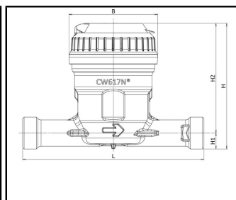
DN 20 - mosiądz
