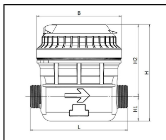
DN 15 - kompozyt
