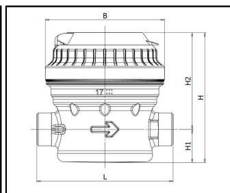
DN 15 - mosiądz
