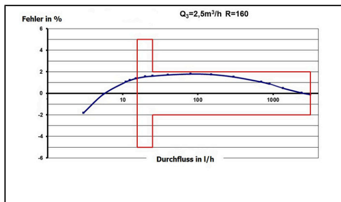
Q_3=2,5 R160
